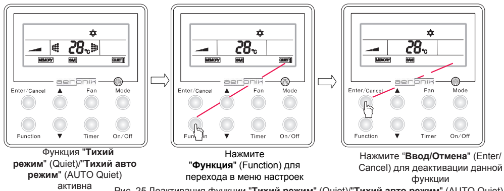
Рис. 25 Деактивация функции "Тихий режим" (Quiet)/"Тихий авто режим" (AUTO Quiet)
